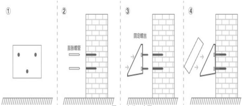
图 1：安装示意图
